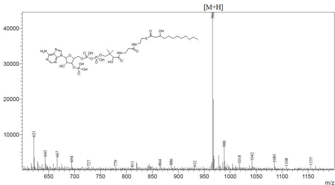
质谱
